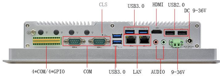
底部I/O视图
