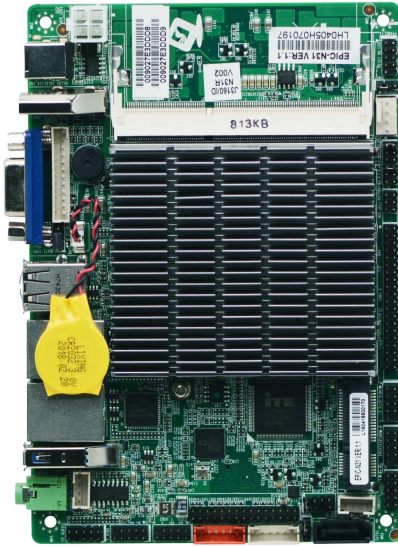
EPIC-N31 主板正面图
