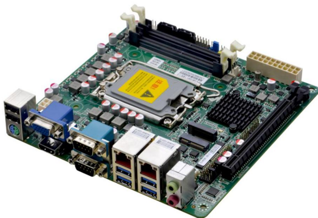
ITX-H610M1 VER:1.0 主板侧面图
