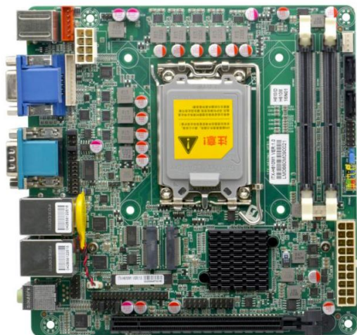
ITX-H610M1 VER:1.0 主板正面图
