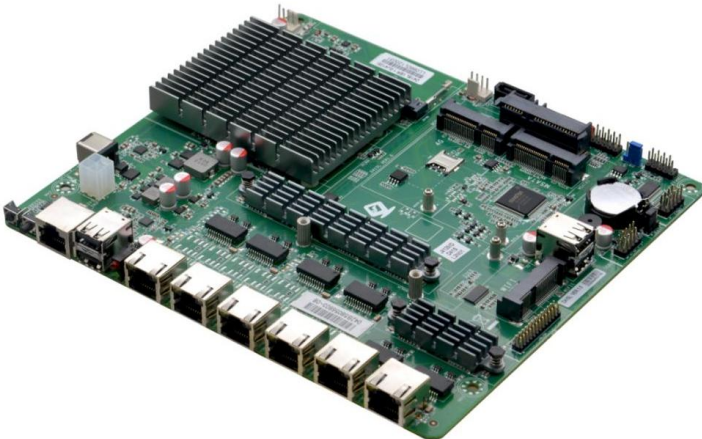
D41SL VER:1.0 主板侧面图
