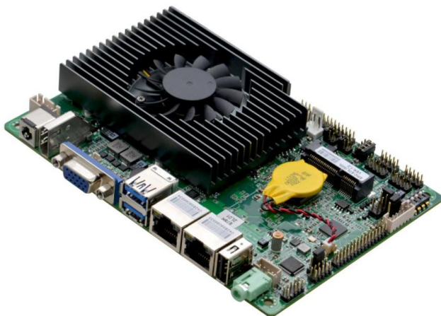
EPIC-E75_I522L VER:1.0 主板侧面图
