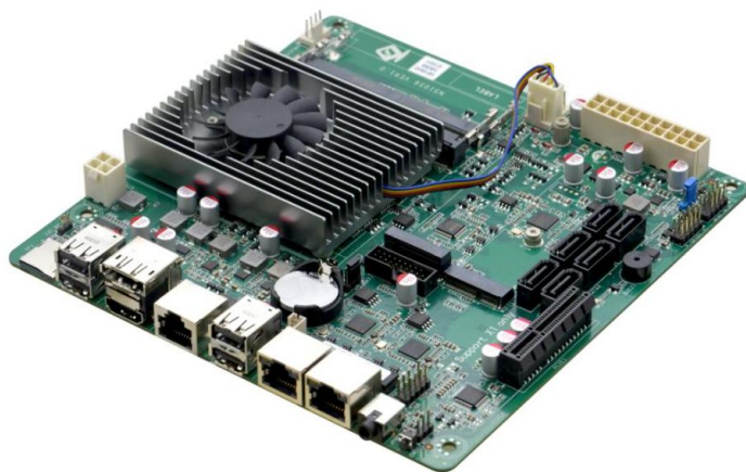
N510S6 VER:1.0 主板侧面图
